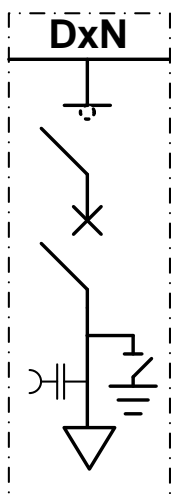
DxN = Disjoncteur
