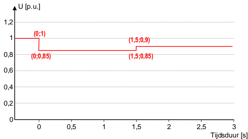
Figuur 13 – Spanning-tijd-profiel voor een noodvoedingssysteem
