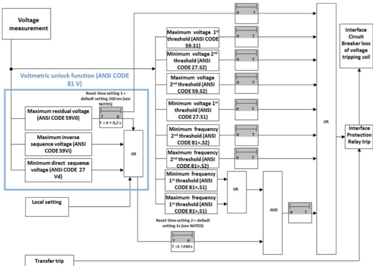
Figuur 7 - Principeschema voor een eilanddetectiefunctie met activering van een nauwer frequentievenster op basis van lokale spanningscriteria (bron: EN50549-1:2019 en EN50549-2:2019)
